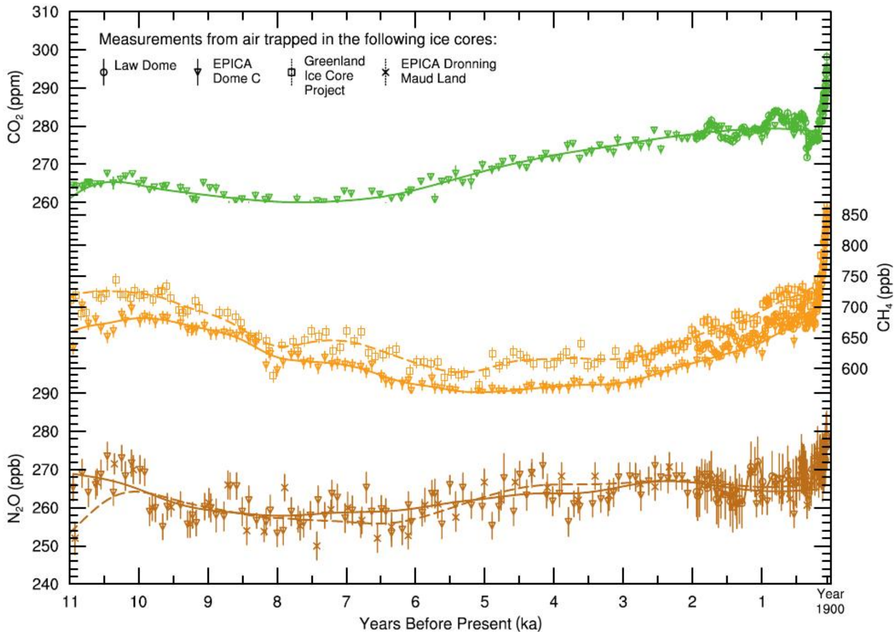
Zmiany w koncentracji atmosferycznych CO 2 , CH 4 i N 2 O w Holocenie.
