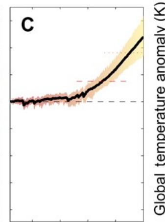
B,C: Globalne anomalie temperatur, najlepsze dopasowanie i zakres niepewności
