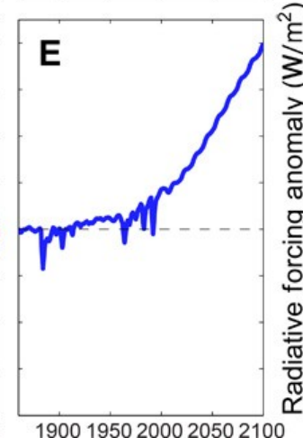
D,E: Wymuszeniaa radiacyjne, których suma jest odpowiedzialna za zmiany temperatury glob. Suma wymuszeń radiacyjnych: linia niebieska
